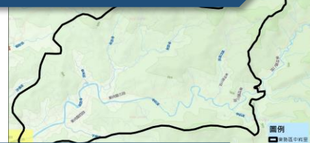
坡地崩塌
